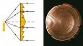
Lentilles Fresnel
